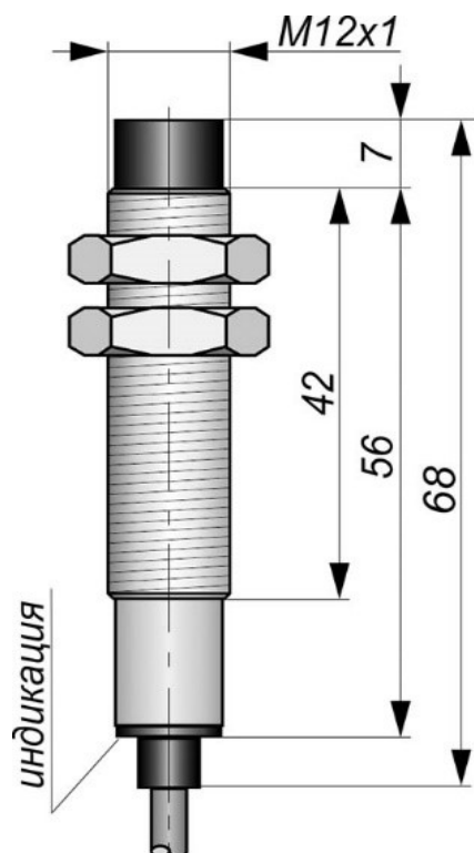
Габаритный чертеж
