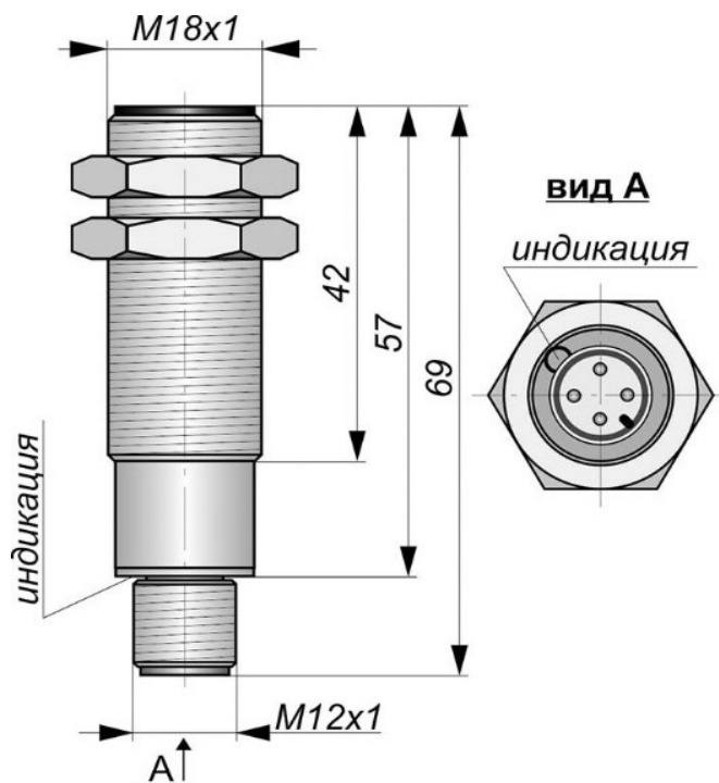
Габаритный чертеж
