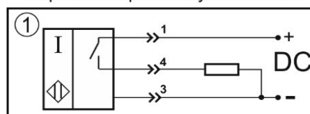
Цоколевка разъема
