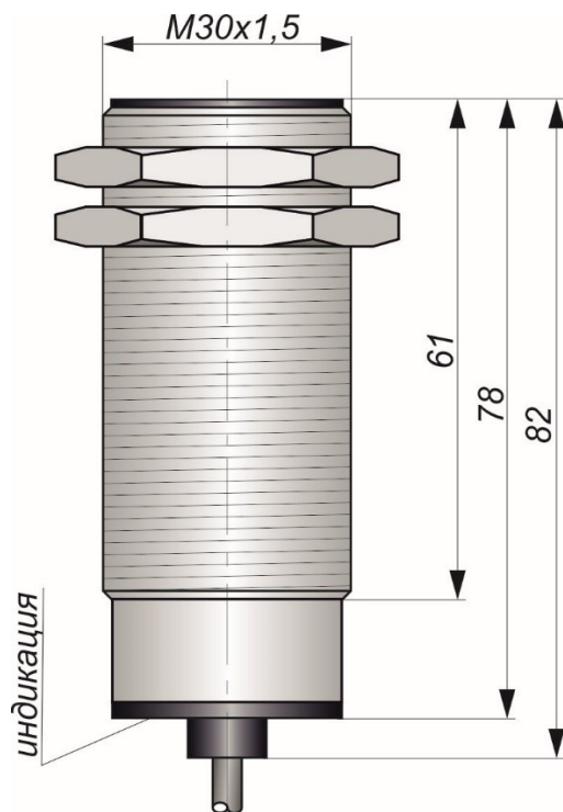
Габаритный чертеж
