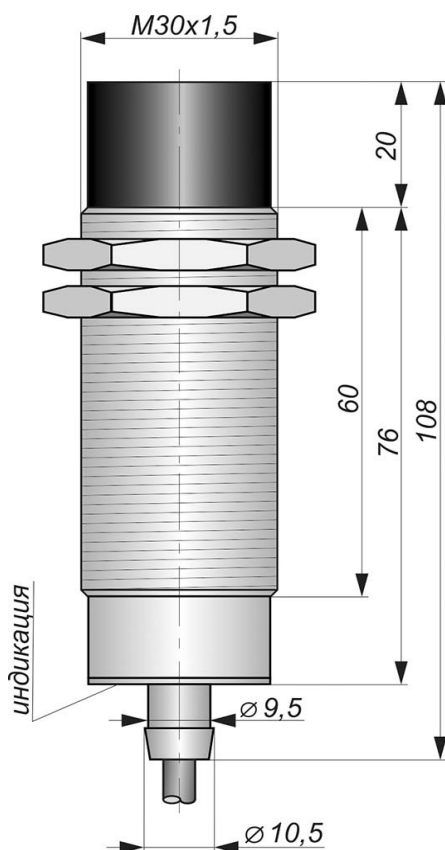
Габаритный чертеж
