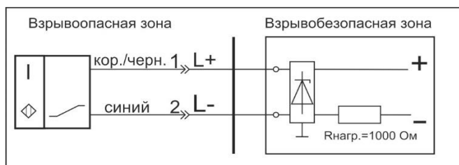
Схема соединения
