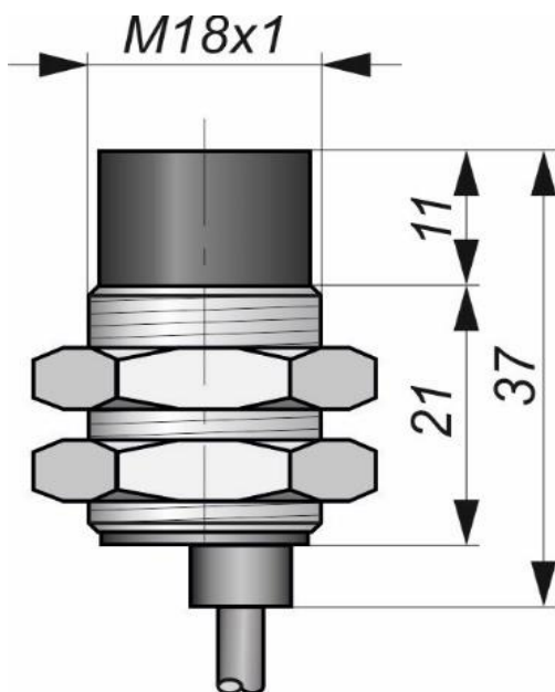
Габаритный чертеж
