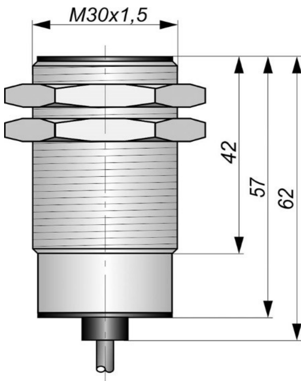
Габаритный чертеж
