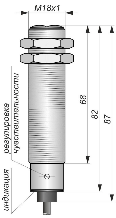
Габаритный чертеж
