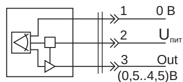
Схема присоединения
