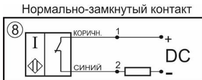
Схема соединения
