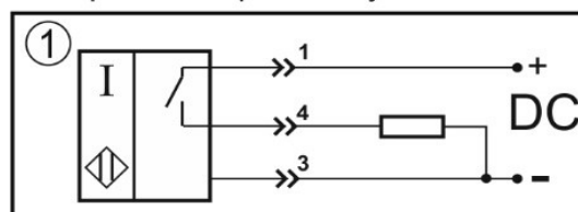
Нормально-разомкнутый контакт
