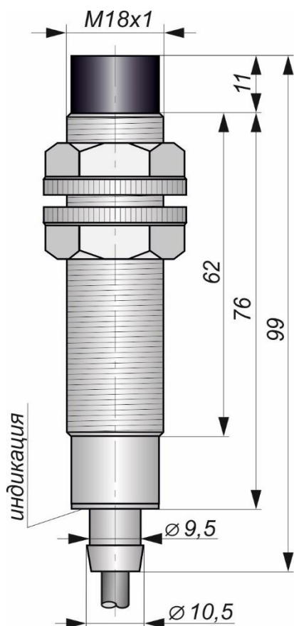
Габаритный чертеж
