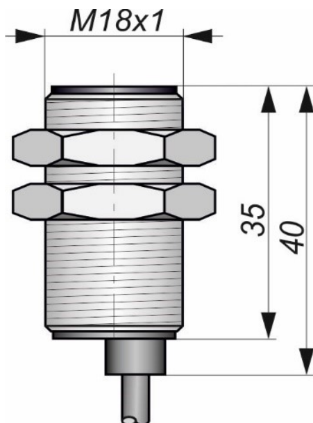
Габаритный чертеж
