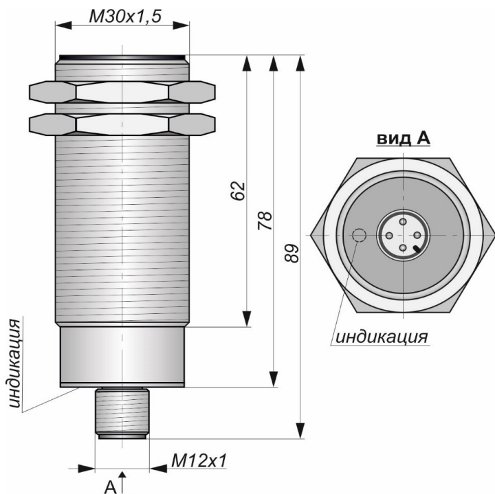
Габаритный чертеж
