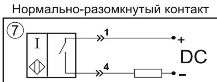
Схема соединения
