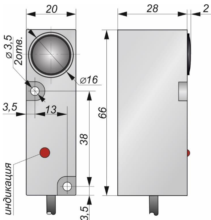
Габаритный чертеж
