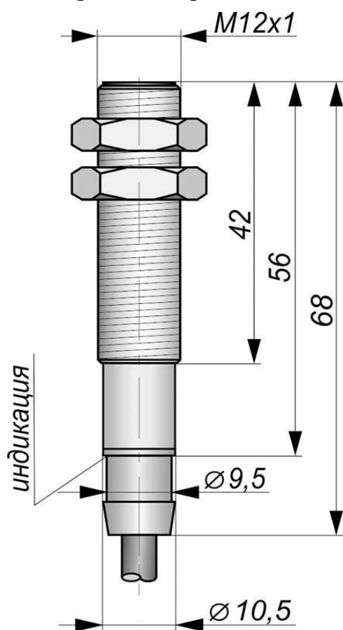
Габаритный чертеж
