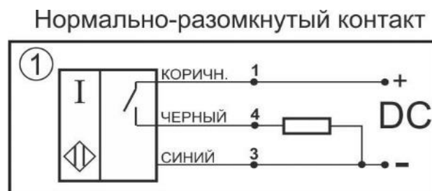
Схема соединения
