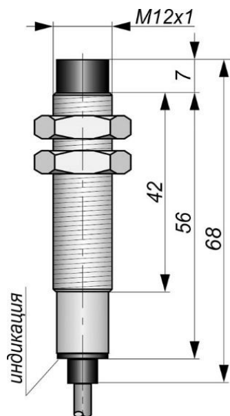
Габаритный чертеж
