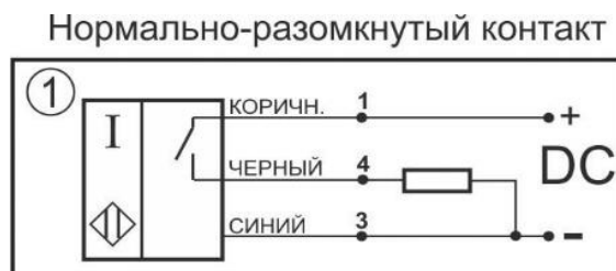
Схема соединения
