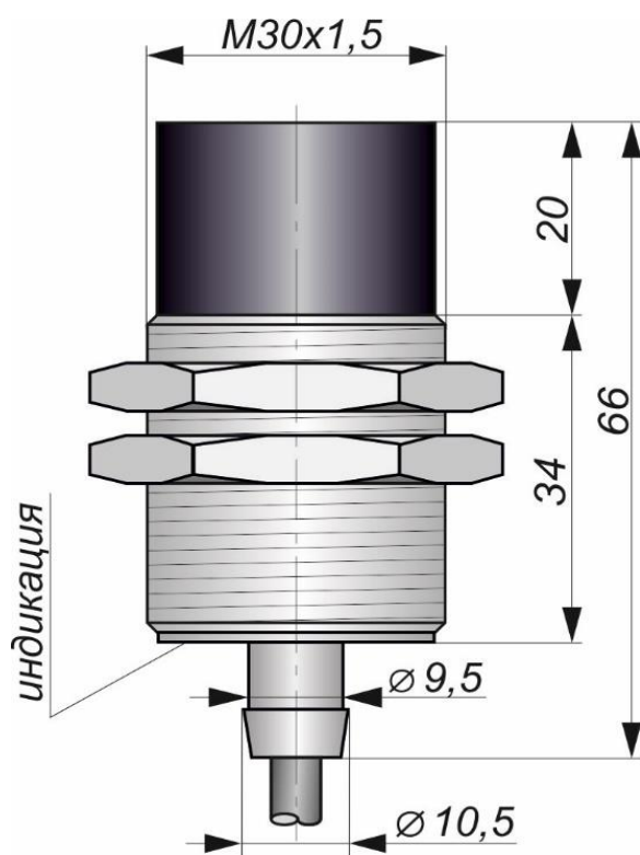
Габаритный чертеж
