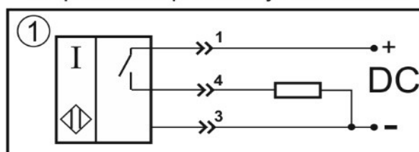
Нормально-разомкнутый контакт
