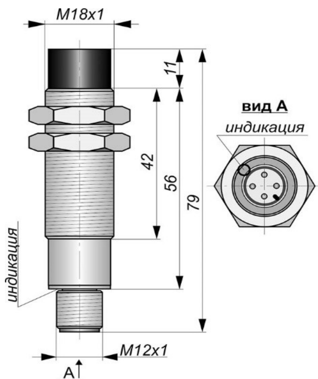
Габаритный чертеж
