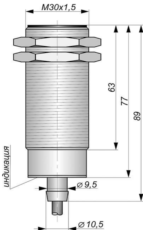
Габаритный чертеж
