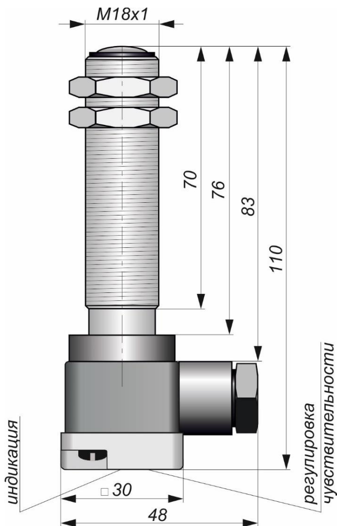
Габаритный чертеж
