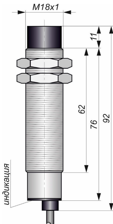
Габаритный чертеж
