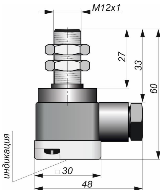
Габаритный чертеж
