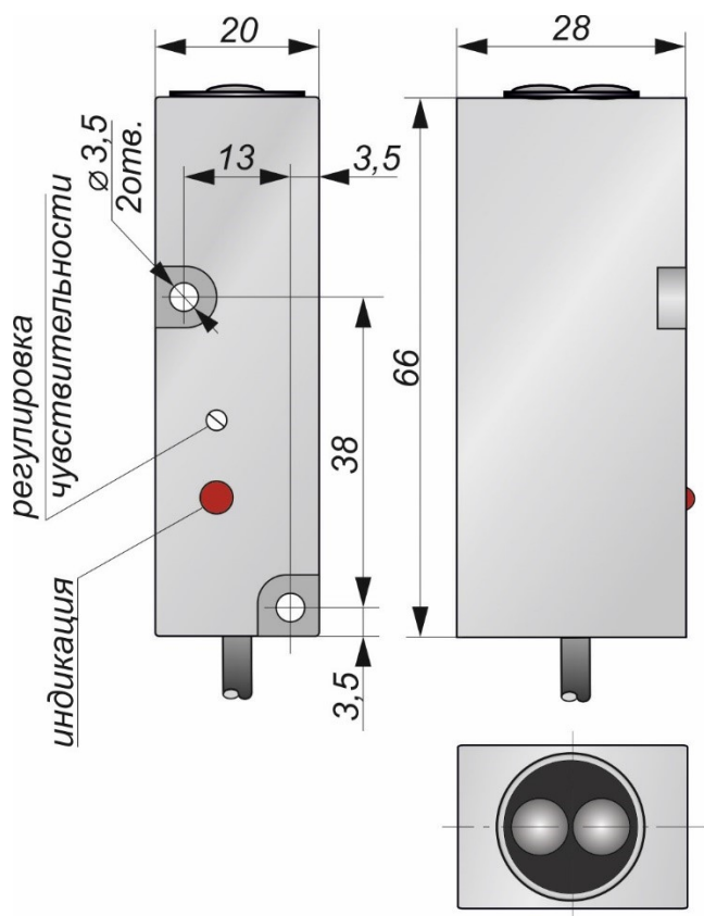
Габаритный чертеж
