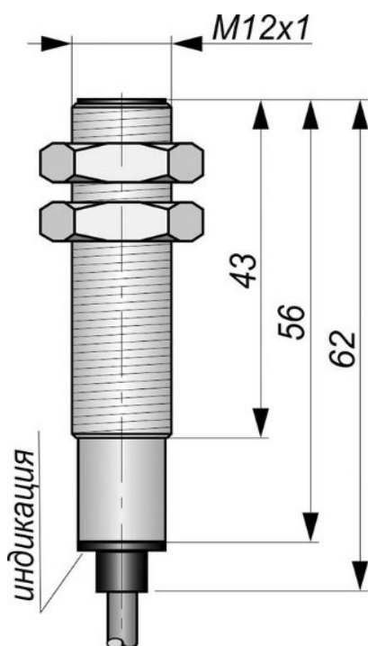
Габаритный чертеж
