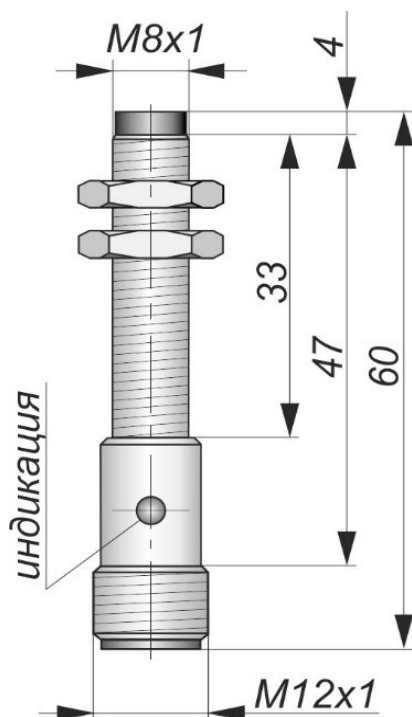
Габаритный чертеж
