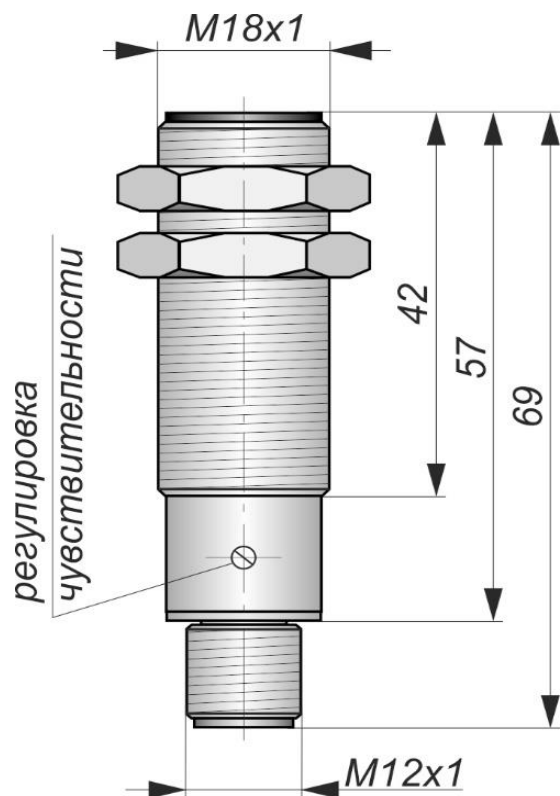
Габаритный чертеж
