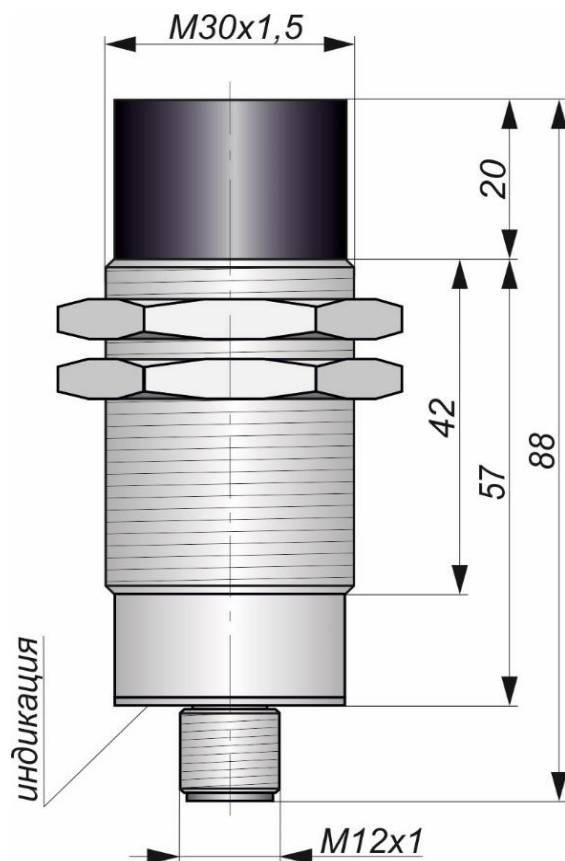
Габаритный чертеж
