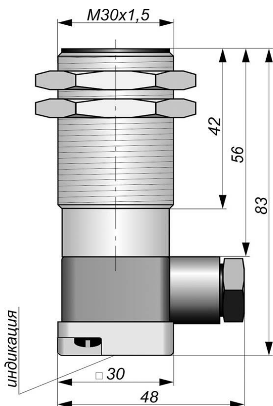
Габаритный чертеж
