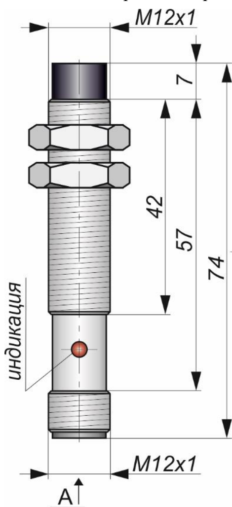
Габаритный чертеж
