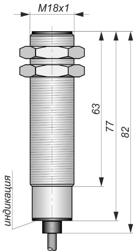
Габаритный чертеж
