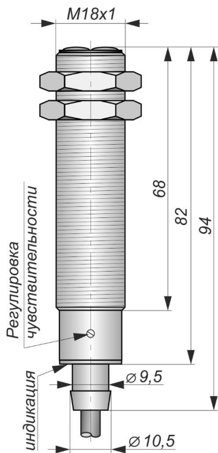
Габаритный чертеж
