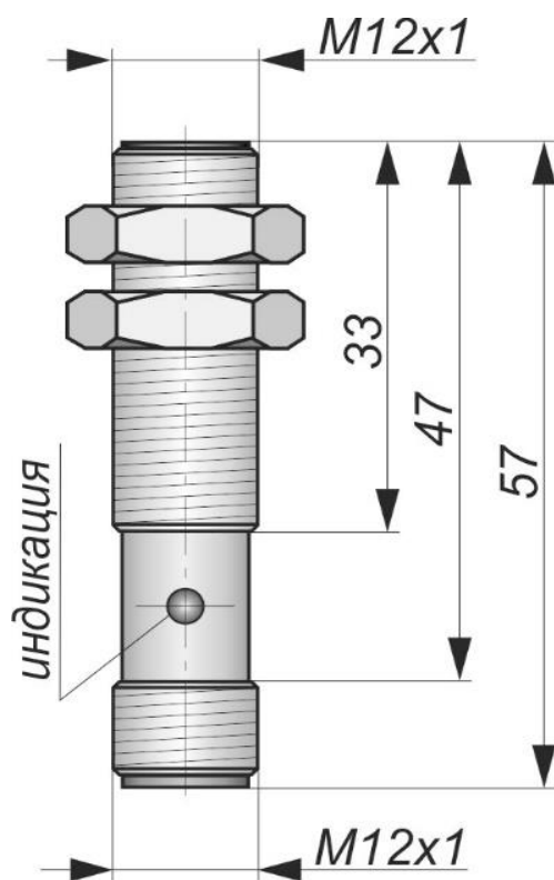
Габаритный чертеж
