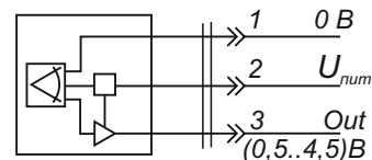
Схема подключения
