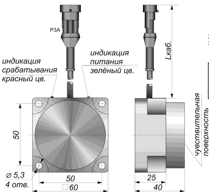
Габаритный чертеж
