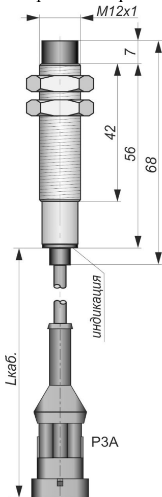
Габаритный чертеж
