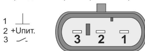
Схема соединения
