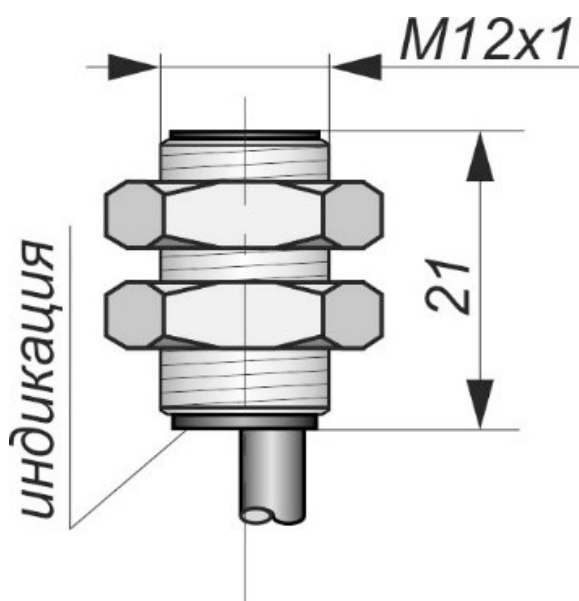
Габаритный чертеж
