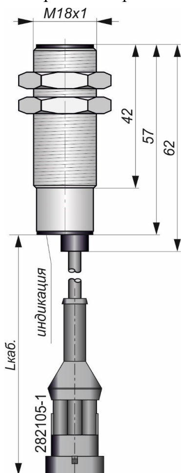
Габаритный чертеж
