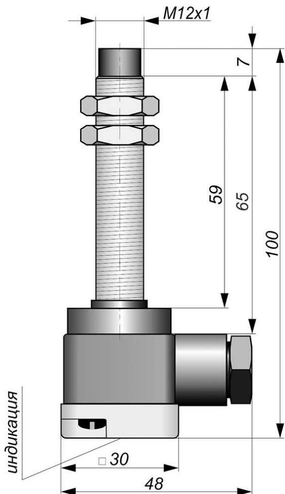
Габаритный чертеж
