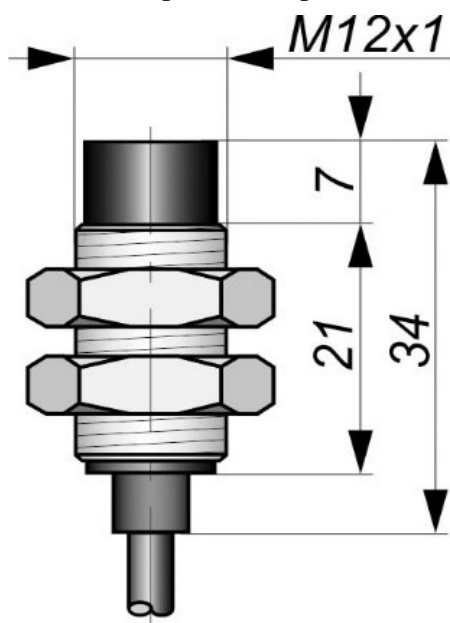
Габаритный чертеж
