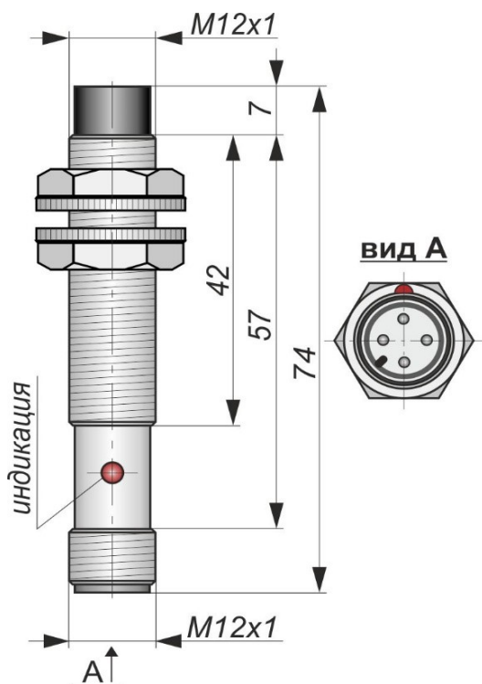
Габаритный чертеж
