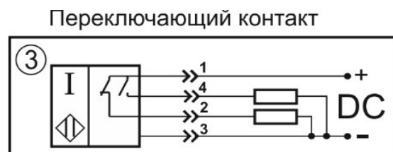
Схема соединения
