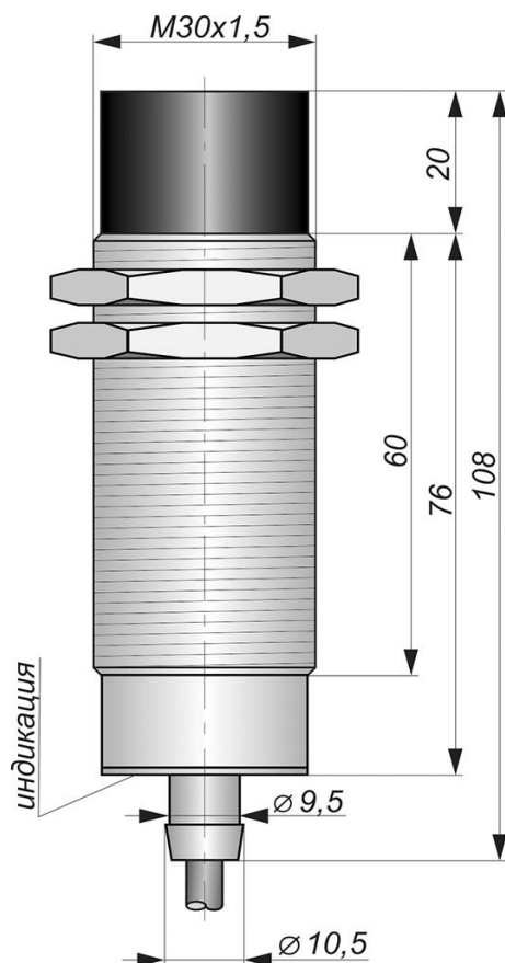
Габаритный чертеж
