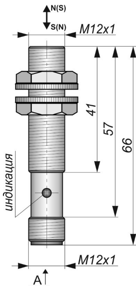
Габаритный чертеж
