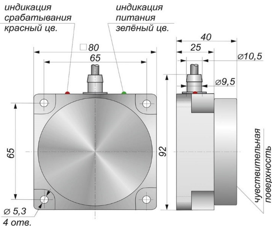
Габаритный чертеж
