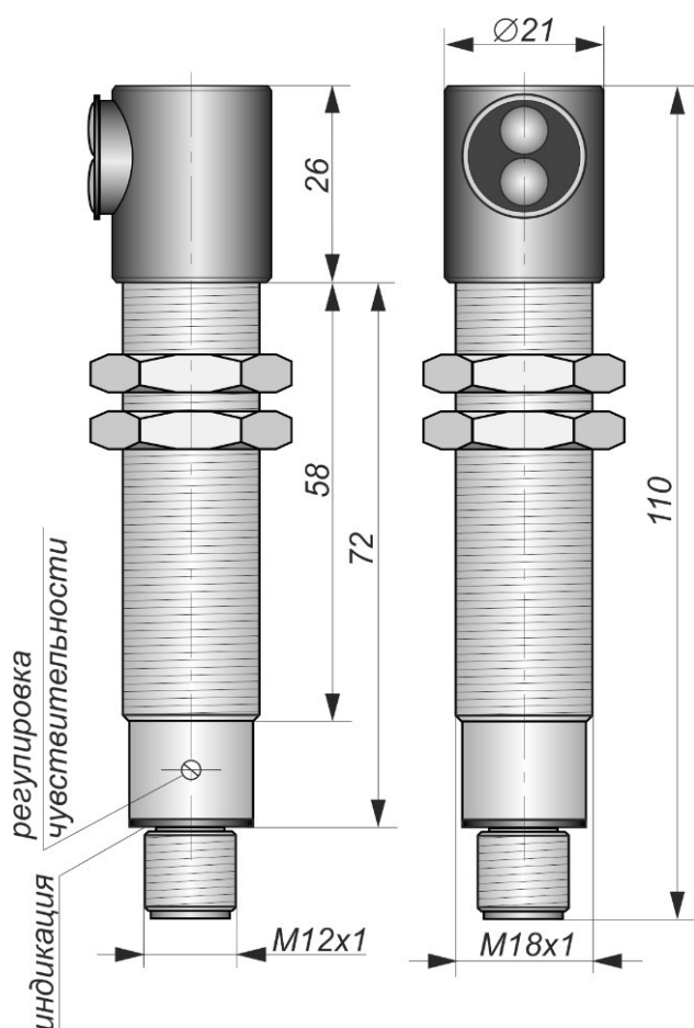
Габаритный чертеж
