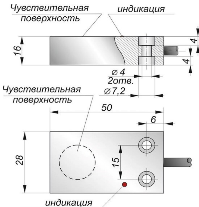
Габаритный чертеж
