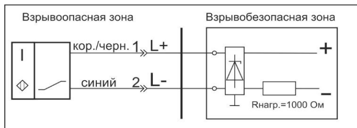
Схема соединения
