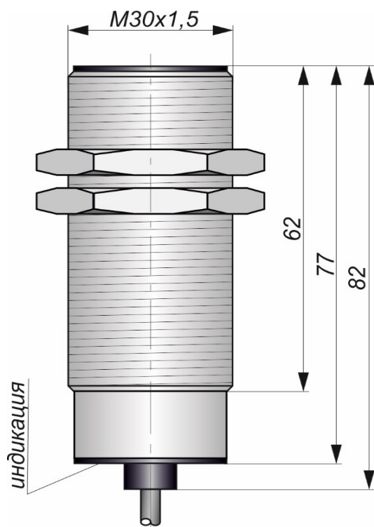
Габаритный чертеж
