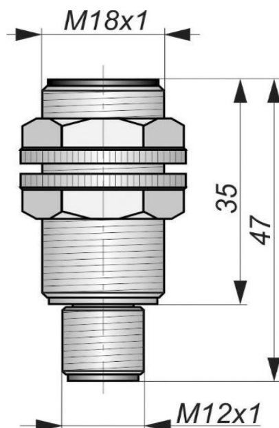
Габаритный чертеж
