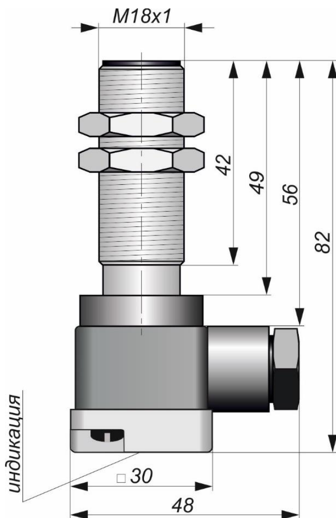
Габаритный чертеж
